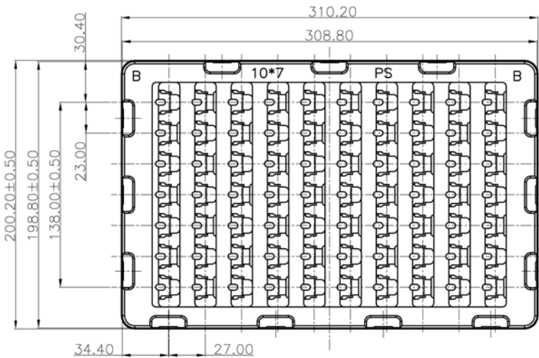
TRAY B LAYOUT SCALE: 1:10
