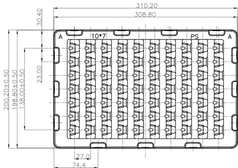
TRAY A LAYOUT SCALE: 1:10
